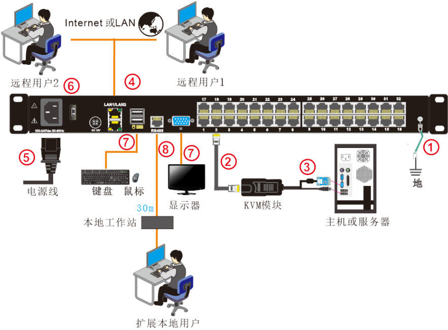
图 2.3 安装示意图
