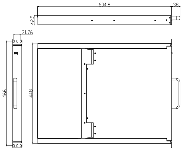
图 1-1.3 19"KVM 尺寸图
