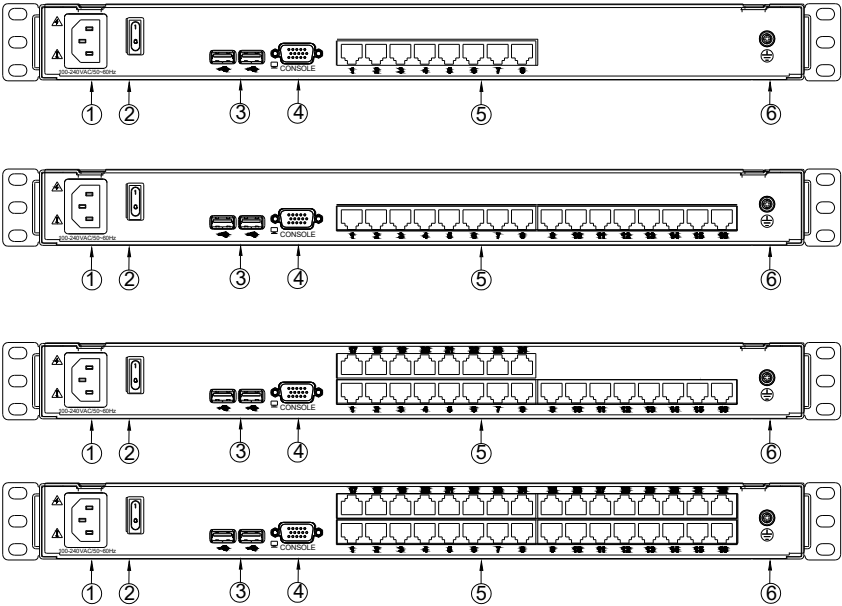
图 1-1.4 后视图
