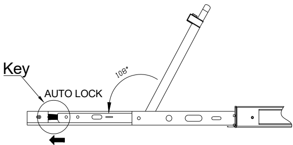
图 2-2.4 控制平台解锁示意图
