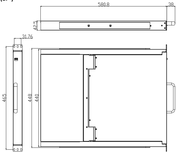
图 1-1.2 17"KVM 尺寸图
