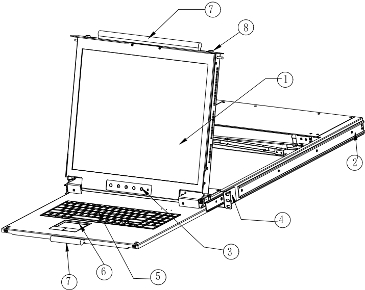
图 1-2 前视图
