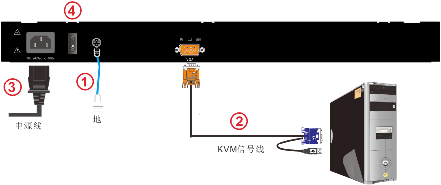
连接图
