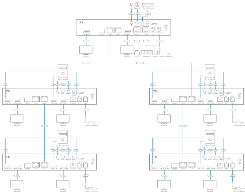
矩阵连接示意图
