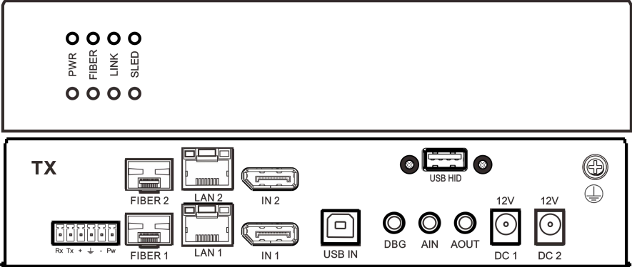
KFP286K 发送端(TX)
