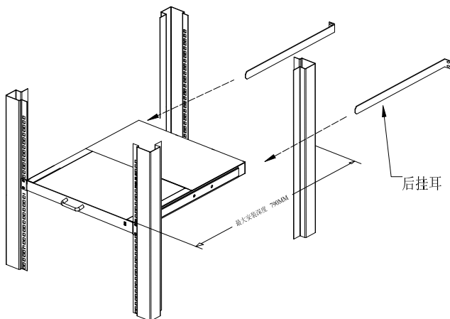
图 2-1 机架安装图(一)
