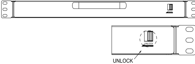
图 2-3 解锁方式
