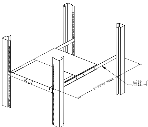
图 2-2 机架安装图(二)
