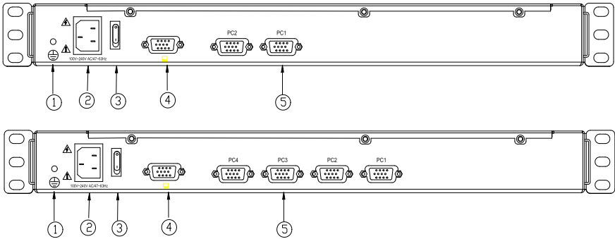
图 1-3 后视图
