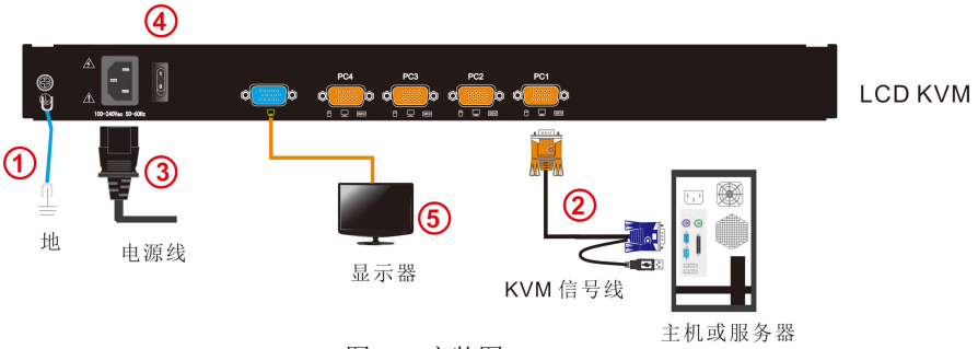
图 1-4 安装图
