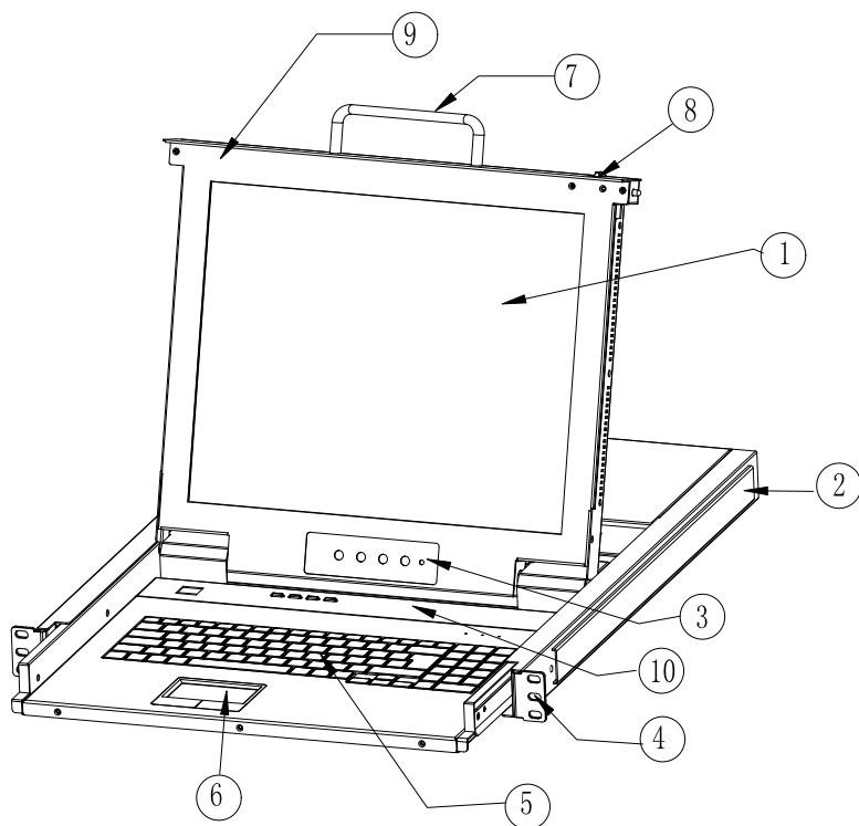
图 1-1 前视图
