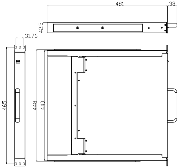
图 1-2 尺寸图
