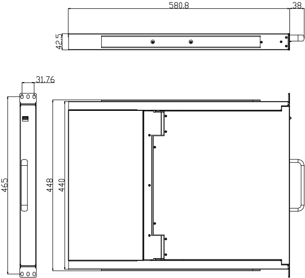
图 1-1.2 17"KVM 尺寸图
