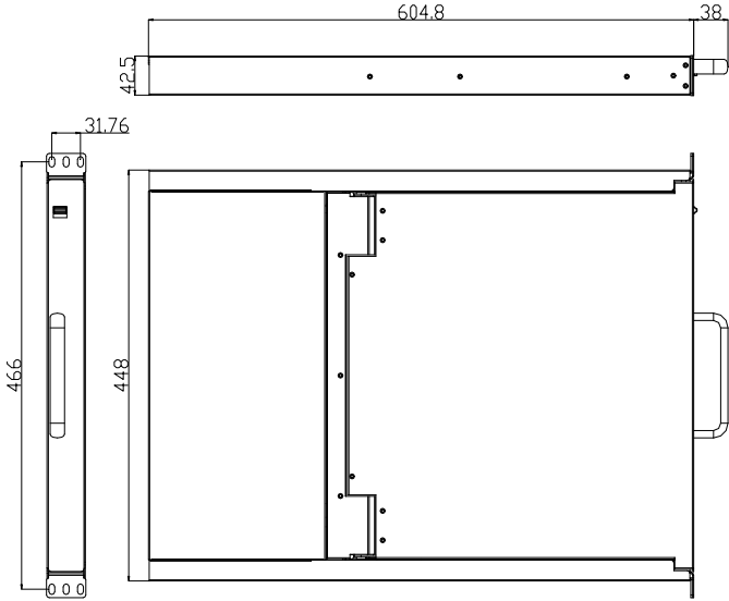
图 1-1.3 19"KVM 尺寸图
