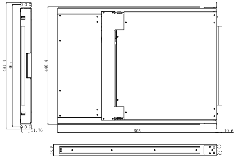
图 1-1.2 尺寸图
