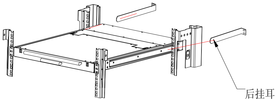
图 1-2.1 机架安装图(一)
