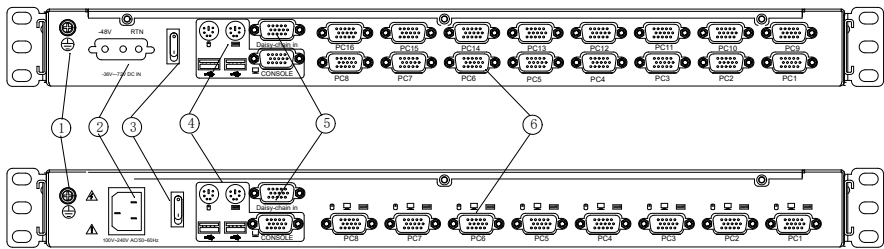
图 1-1.3 后视图
