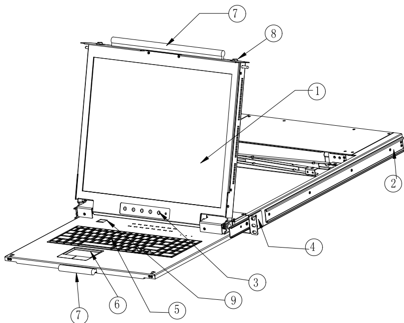
图 1-1.1 前视图
