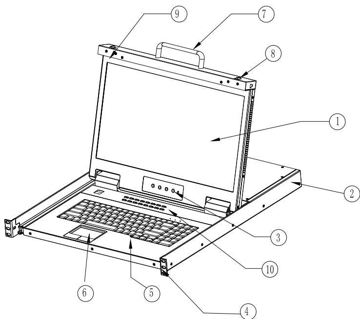
图 1-1.1 前视图
