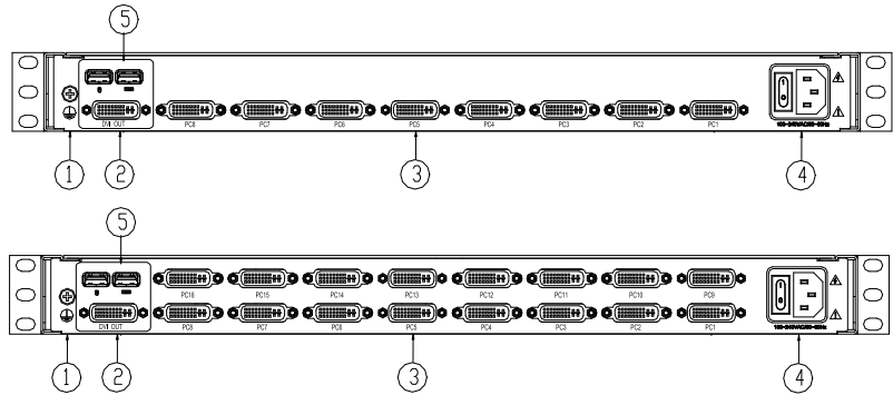
图 1-1.3 后视图
