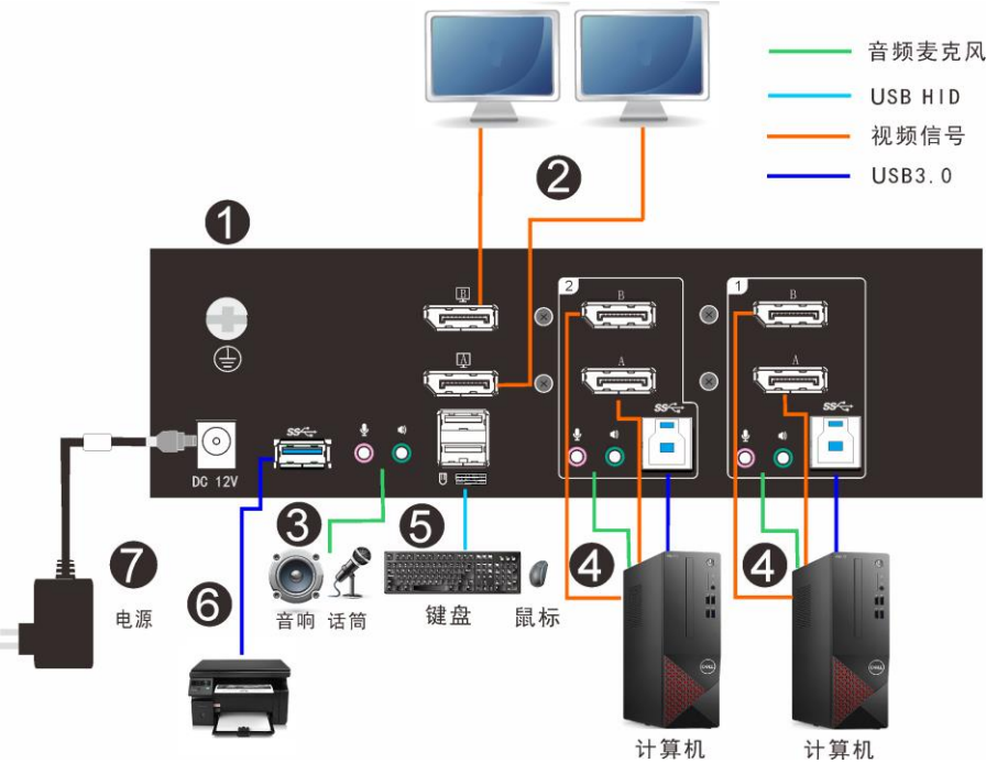
连接示意图
