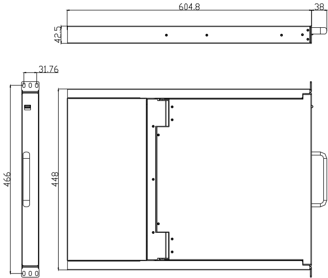
图 1-3 19"尺寸图
