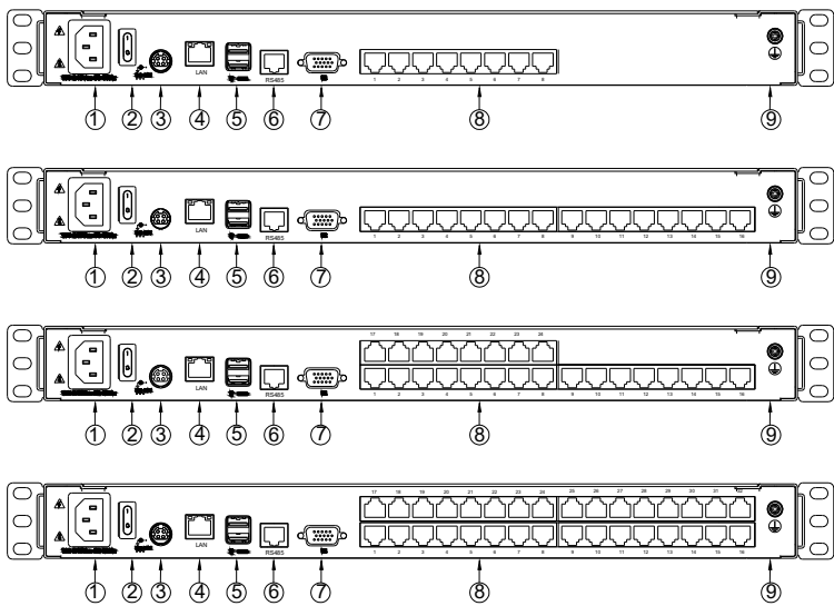
图 1-4 后视图
