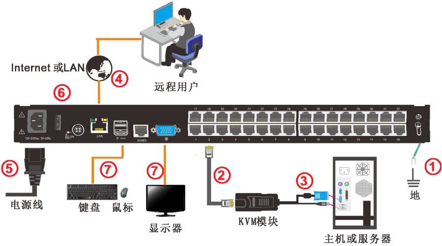
图 2-3 安装示意图
