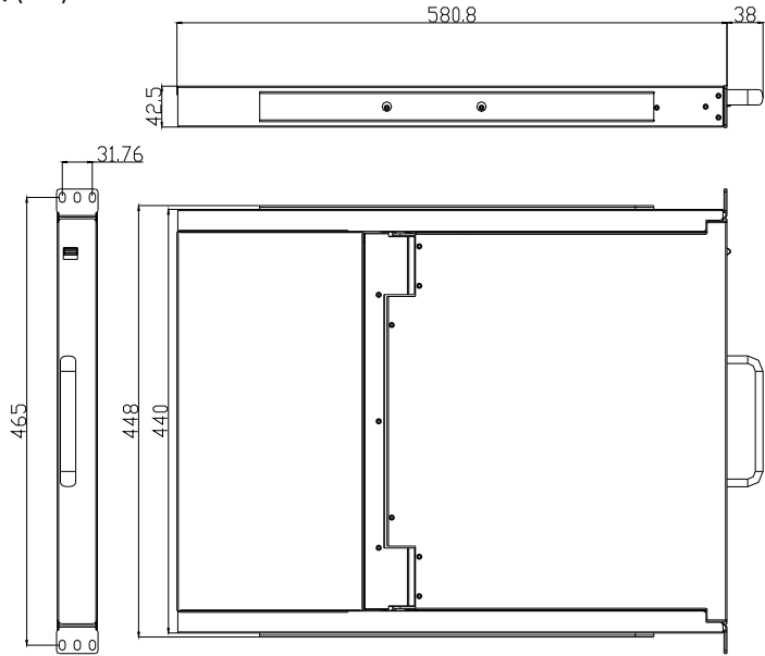
图 1-2 17"尺寸图
