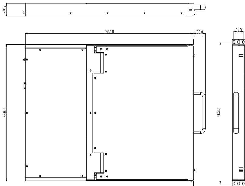
图 1-1.2 尺寸图
