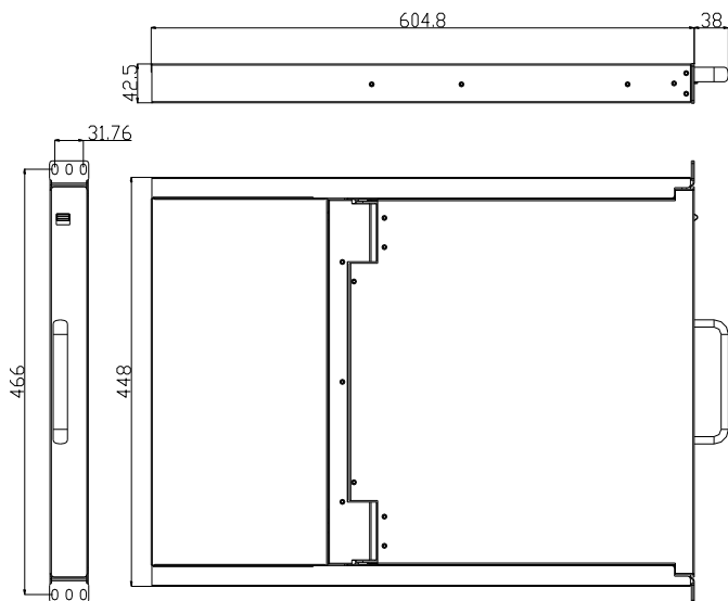
图 1-1.3 19"KVM 尺寸图
