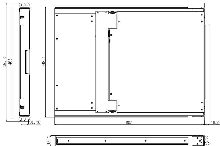
图 1-1.2 尺寸图
