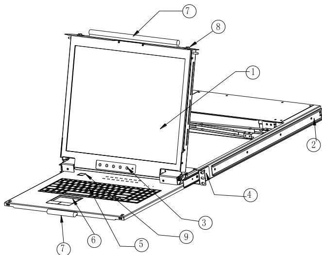
图 1-1.1 前视图
