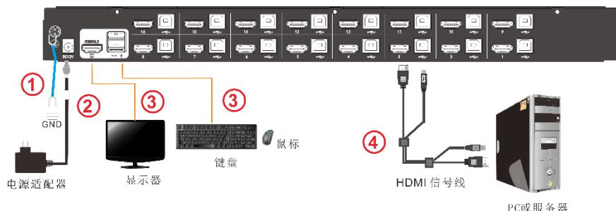
图 1.2 安装 KVM 配件图
