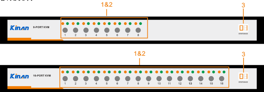
图 1.3 KVM 前视图
