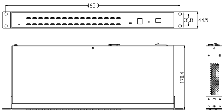
图 1-1.2 尺寸图
