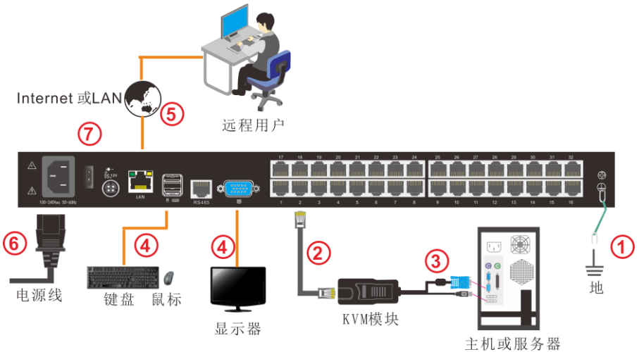
图 2-2.1 安装示意图
