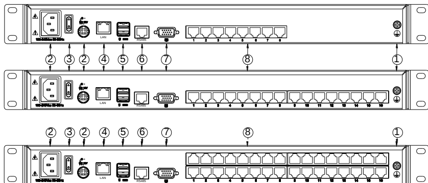
后视图
