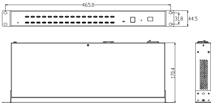
图 1-1.2 尺寸图
